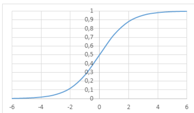
Рис. 1 – График логистической функции
